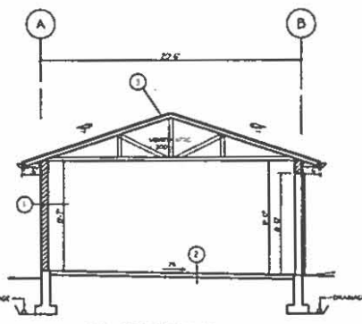
8 SECTION B SCALE: 1/4" = 1'-0"
