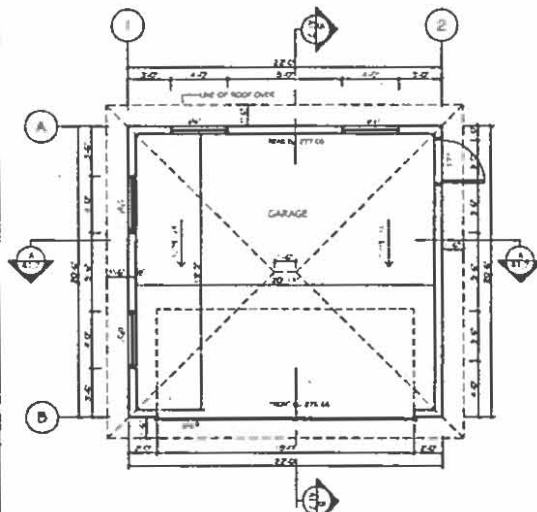
1 FLR PLAN SCALE: 1/4" = 1'-0"
