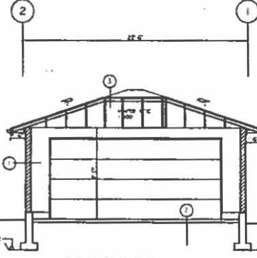
7 SECTION A SCALE: 1/4" = 1'-0"
